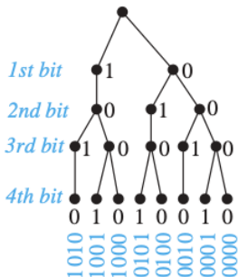
Figura 4: Cadenas de longitud cuatro sin dos unos consecutivos.
