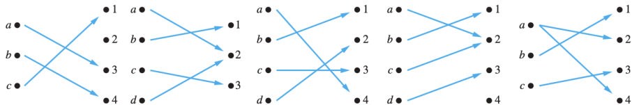
Figura 5: Ejemplos de diferentes tipos de correspondencias.
