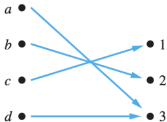
Figura 4: Una función sobre.
