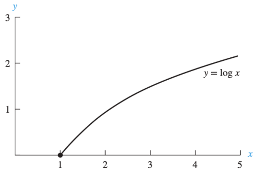
Figura 12: La gráfica de f(x) = \log x .
