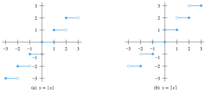
Figura 10: Las gráficas de las funciones (a) piso y (b) techo.
