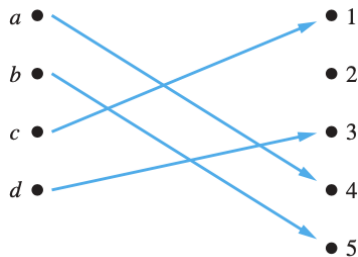
Figura 3: Una función uno a uno.
