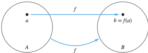
Figura 2: La función f mapea A en B .
