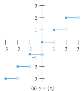
Figura 10: Las gráficas de las funciones (a) piso y (b) techo.
