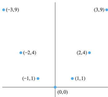
Figura 9: La gráfica de f(x) = x^2 de \mathbb{Z} a \mathbb{Z} .
