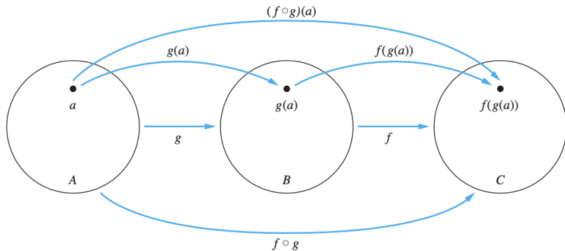
Figura 7: La composición de las funciones f y g .
