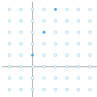
Figura 8: La gráfica de f(n) = 2n + 1 de \mathbb{Z} a \mathbb{Z} .
