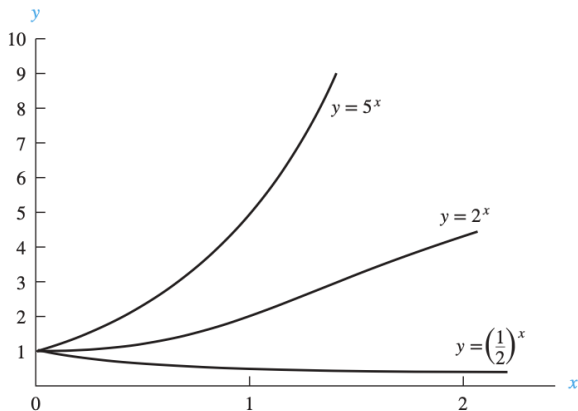
Figura 11: Gráficas de las funciones exponenciales en bases \frac{1}{2} , 2 y 5.
